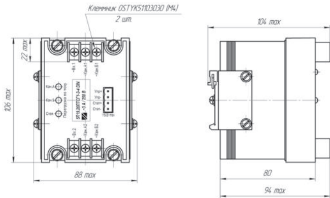
Габаритный чертеж
