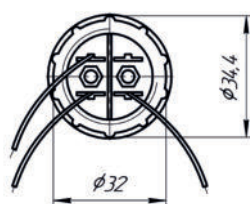
табачный чертёж двухцветной СКЛ11
