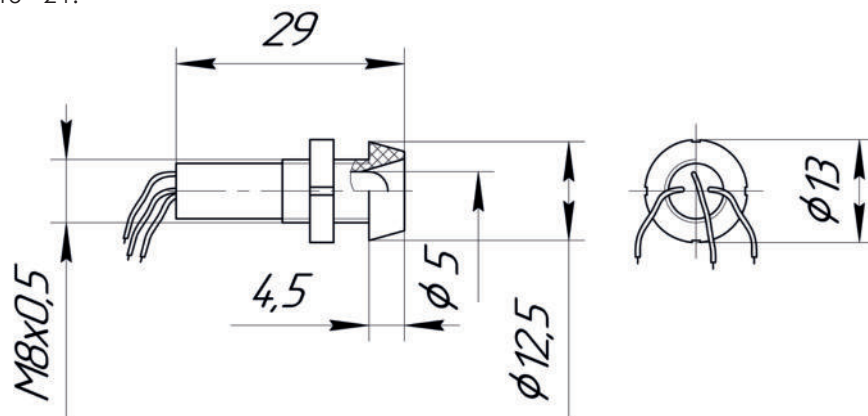
габаритный чертёж двухцветной СКЛ15 (исполнение в пластмассовом корпусе)
