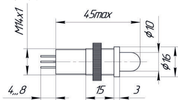
габаритный чертеж двухцветной СКЛ18 (исполнение в пластмассовом корпусе)
