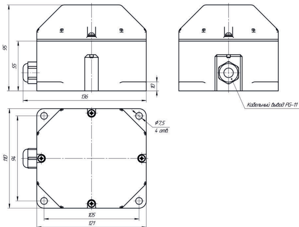
Габаритный чертеж
