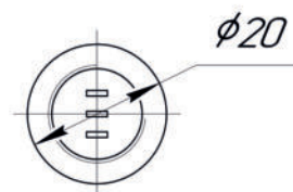
габаритный чертеж двухцветной СКЛ18 (исполнение в пластмассовом корпусе)
