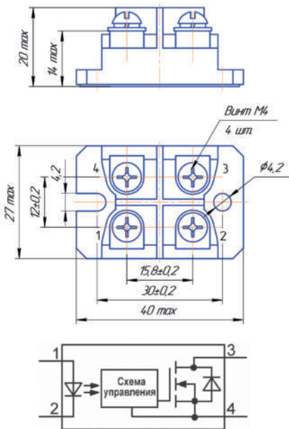
Габаритный чертёж
