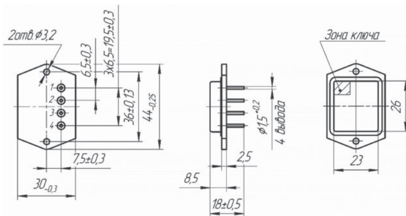
Габаритный чертеж
