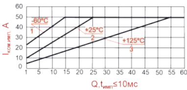
Типовая зависимость импульсного коммутируемого тока I_{\text{ком.имп.}} от скажности импульса Q в диапазоне температур корпуса
