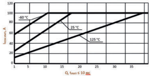
Область безопасной работы - не выше границы. Зависимость импульсного коммутируемого тока I_{ком.имп} от скважности импульса Q в диапазоне температур корпуса
