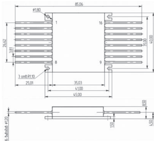
Габаритный чертёж
