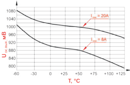
Типовая зависимость выходного постоянного напряжения в открытом состоянии U_{ос.вых.} от температуры корпуса и коммутируемого тока I_{ком.}
