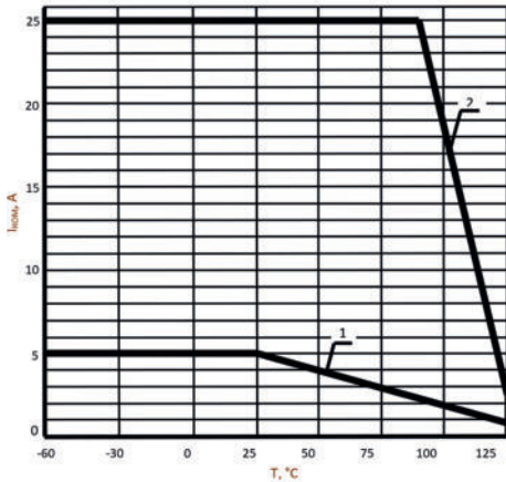
1 - без теплоотвода; 2 - с теплоотводом 1,12 \text{ } ^\circ\text{C}/\text{Вт} Область безопасной работы - не выше границы. Зависимость предельно-допустимого коммутируемого тока I_{ком} от температуры корпуса
