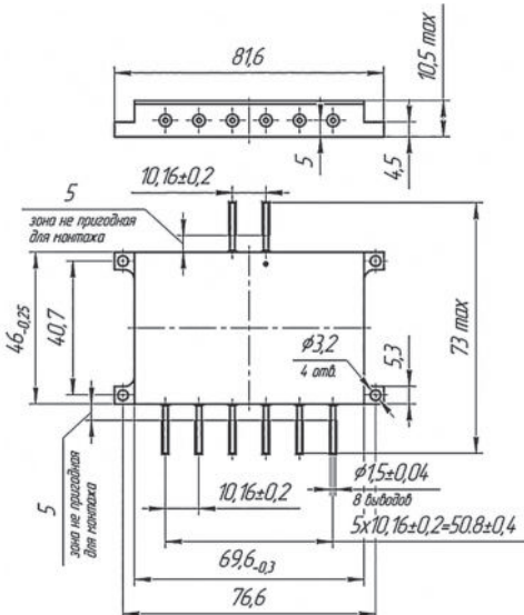
Габаритный чертёж
