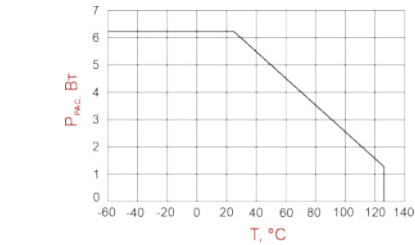
Типовая зависимость рассеиваемой мощности P_{\text{расс.}} от температуры окружающей среды при работе без теплоотвода
