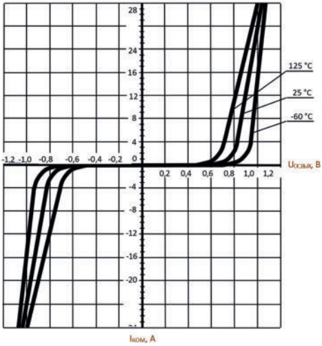
Зависимость выходного постоянного напряжения в открытом состоянии U_{с.вых} от коммутируемого тока I_{ком} в диапазоне температур
