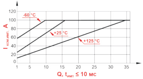
Типовая зависимость импульсного коммутируемого тока I_{ком.имп.} от скважности импульса Q в диапазоне корпуса
