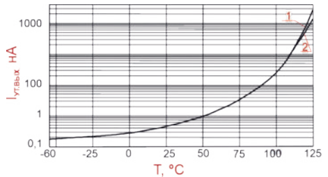
Типовая зависимость тока утечки на выходе I_{\text{ут.вых.}} от температуры корпуса при постоянном напряжении на выходе 100В (диапазон значений)
