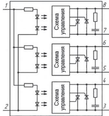
Структурная электрическая схема и функциональное назначение выводов
