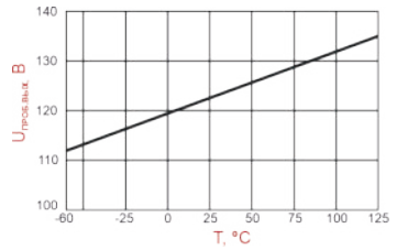
Типовая зависимость напряжения пробоя выхода U_{\text{проб.вых.}} от температуры окружающей среды при I_{\text{проб.вых.}} = 10\text{mA}
