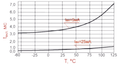
Типовая зависимость времени включения t_{\text{вкл.}} от температуры корпуса в диапазоне входного тока I_{\text{вх}}
