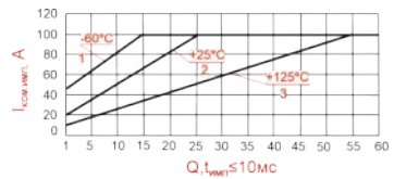
Типовая зависимость импульсного коммутируемого тока I_{\text{ком.имп.}} от скажности импульса Q в диапазоне температур корпуса
