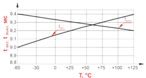
Типовая зависимость времени включения t_{вкл.} и времени выключения t_{выкл.} от температуры корпуса при U_{ком.} = 250В , I_{ком.} = 5А , f_{ком.} = 50Гц
