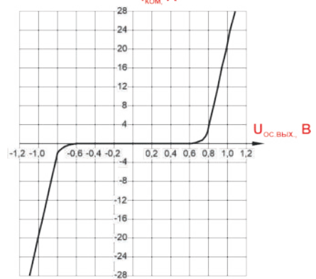
Типовая зависимость напряжения в открытом состоянии U_{ос.вых} от коммутируемого тока I_{ком} при температуре корпуса (25 \pm 10)^\circ C
