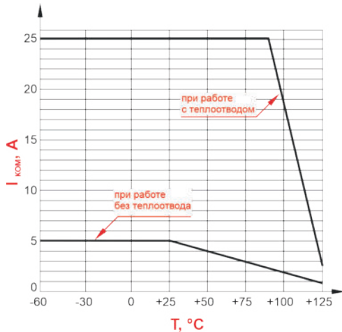
Типовая зависимость предельно допустимого коммутируемого тока I_{ком.п.} от температуры корпуса
