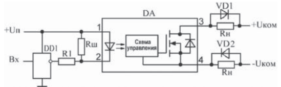
Типовая схема включения
