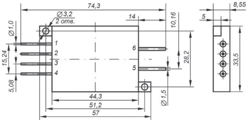
Габаритный чертеж
