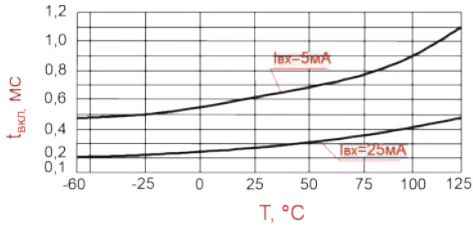
Типовая зависимость времени включения t_{\text{вкл.}} от температуры корпуса в диапазоне входного тока I_{\text{вх}}
