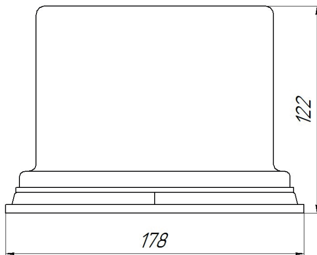
Габариты: 122хØ178мм Количество светодиодов - 6
