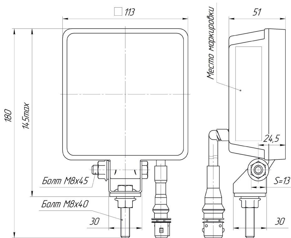
Габаритные и присоединительные размеры фары ●
