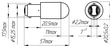
Цоколь BA15d
