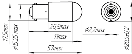
Цоколь B15s
