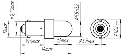
Цоколь BA9s
