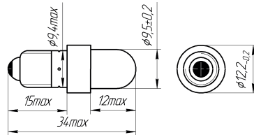
Цоколь E10
