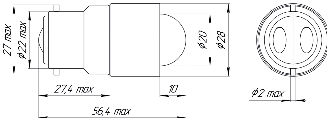
Габаритный чертеж
