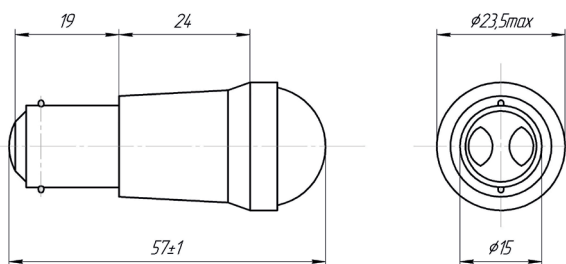
Габаритный чертёж
