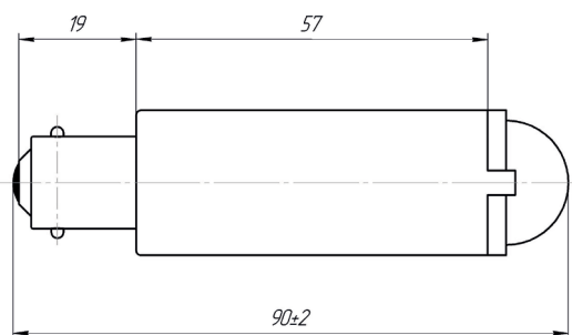
Габаритный чертеж
